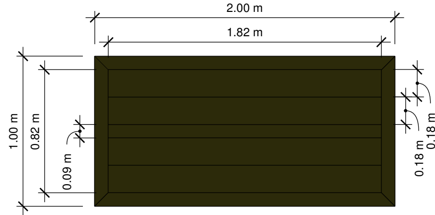
Top Elevation
