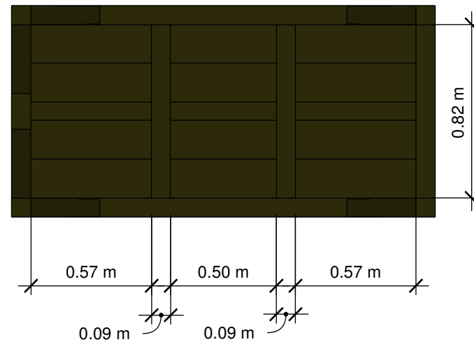
Bottom Elevation
