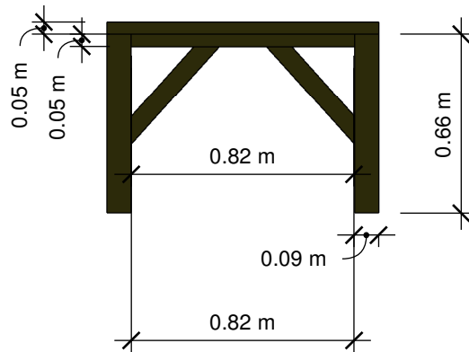
Right Elevation
